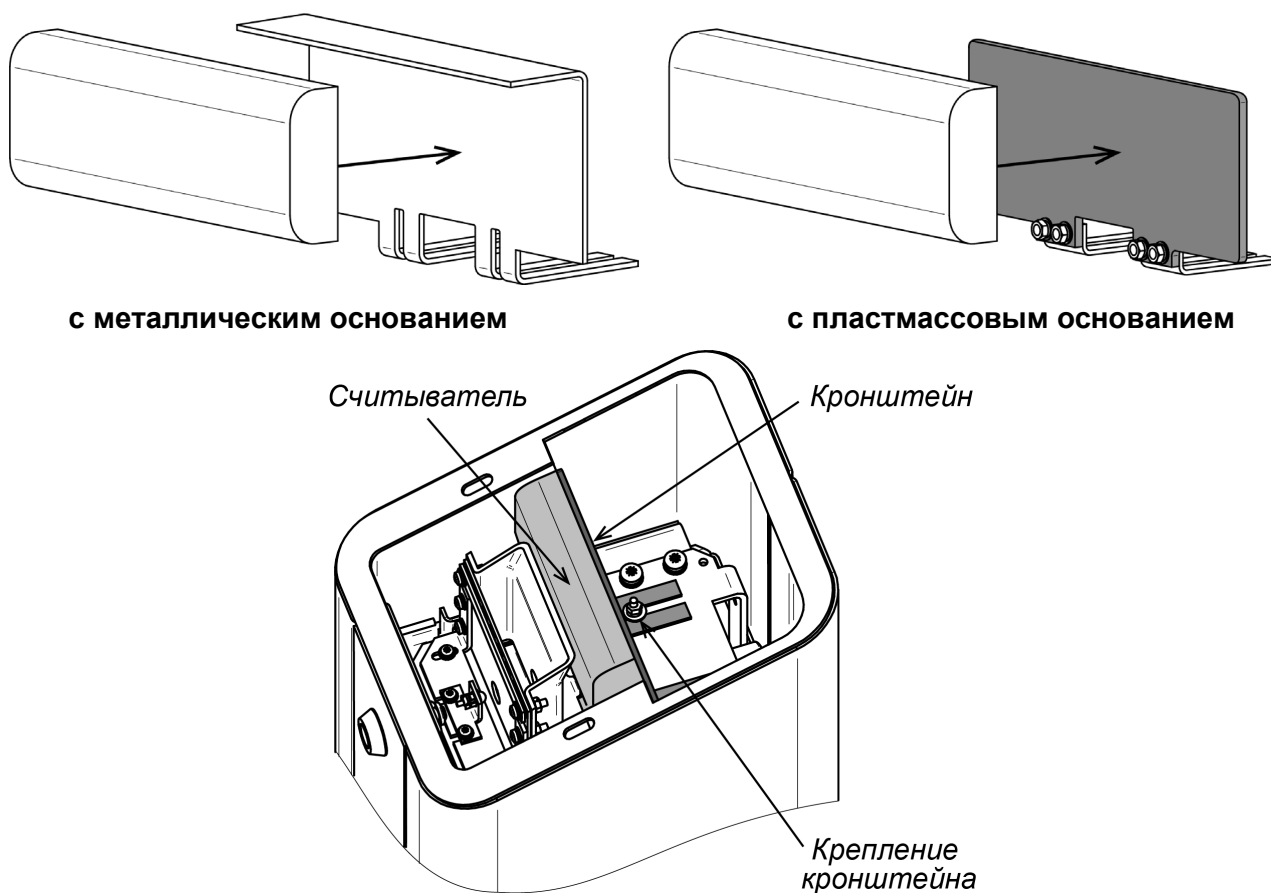
Рисунок 6. Установка считывателя на кронштейн
