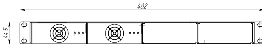
Вид спереди
