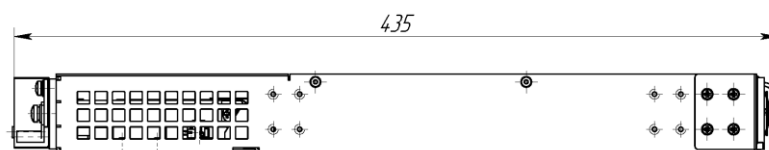
Вид сбоку
