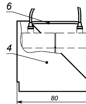
Рис. 1.2 Устройство, габаритные и установочные размеры КБП-24/150 (2,2А·ч) Остальное см. Рис.1.1.
