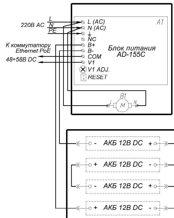
Рис.2.2 Схема электрическая принципиальная КБП-48/150 (2,2 А·ч)
