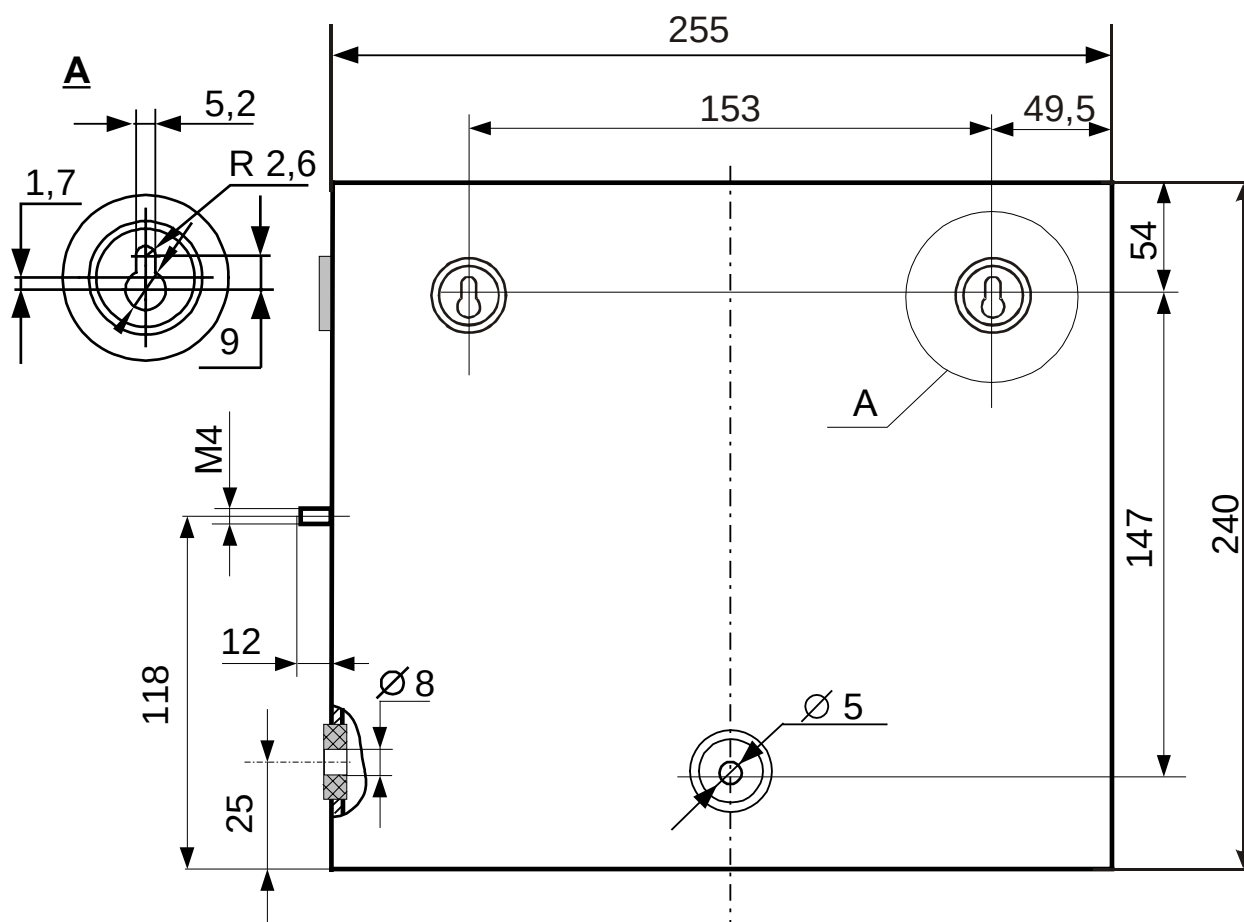
Рис. 12 Габаритные и присоединительные размеры КД2 исп.08-1
