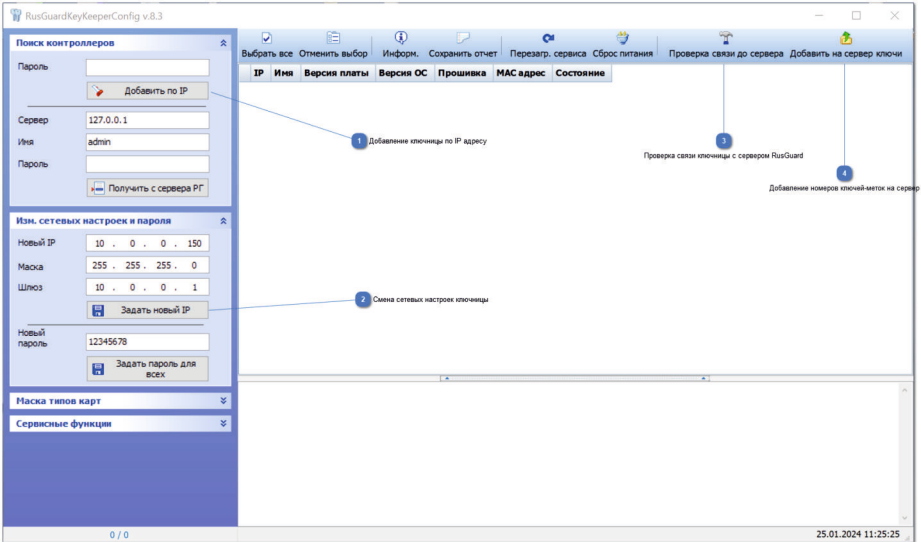
Рис.5 Утилита RusGuardKeyKeeperConfig
