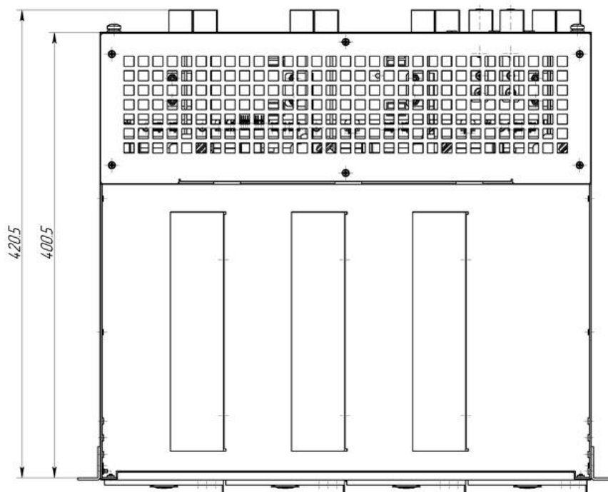
Вид сверху
