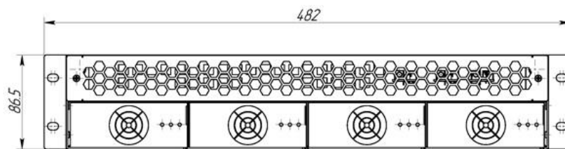
Вид спереди
