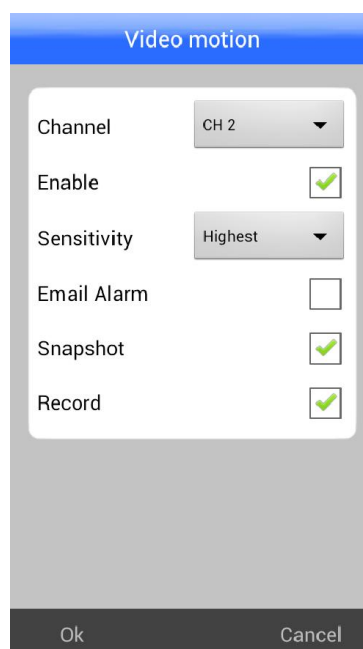
Рис. 7.1.11. Меню Video Motion
