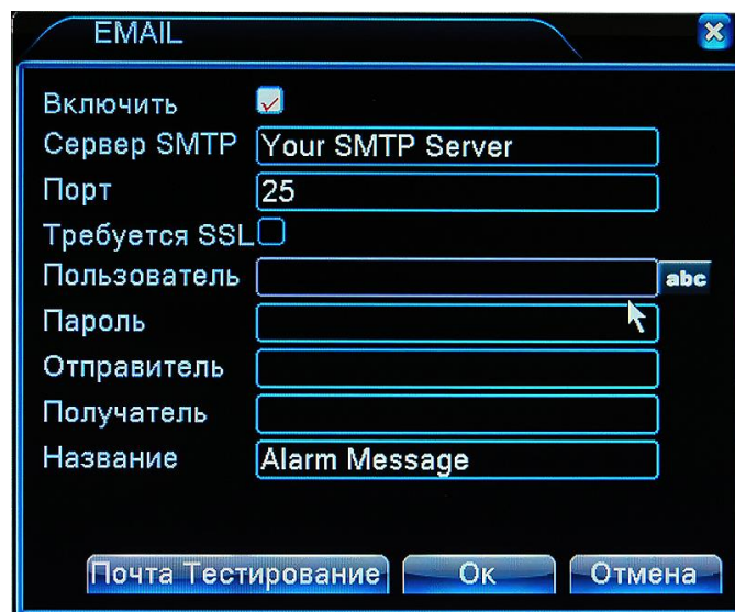
Рис. 4.3.4.4. Настройка. Сетевые службы. E-mail
