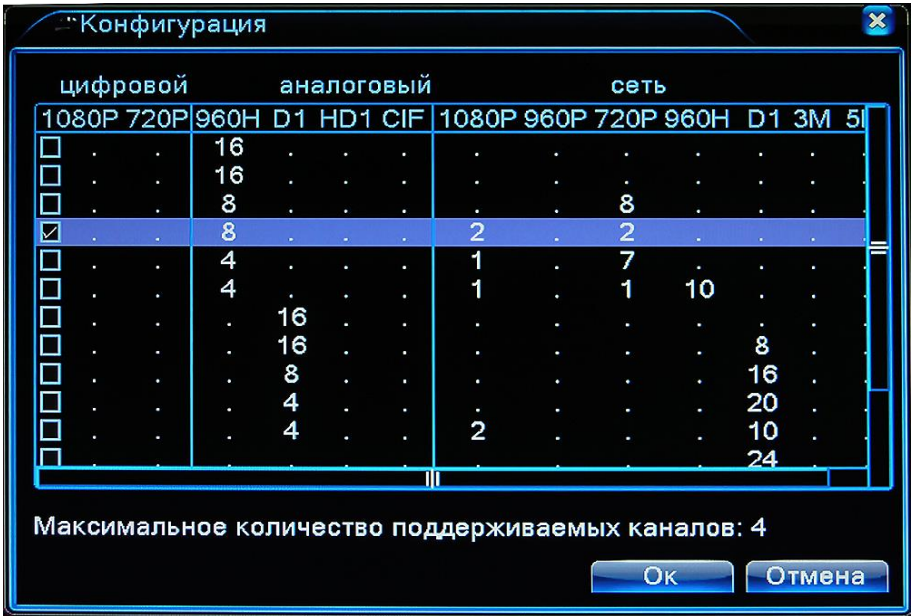
Рис. 4.3.9.2. Главное меню. Настройка. Цифровой. Тип каналов
