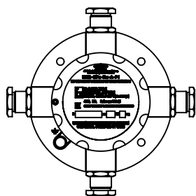
ККВ Р1-00.000-4 Крестовая
