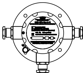
ККВ Р1-00.000-3 Тройниковая
