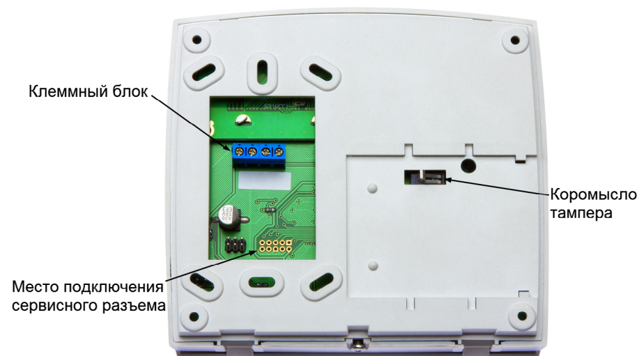
Рисунок 2. Вид клавиатуры АКД-01 сзади
