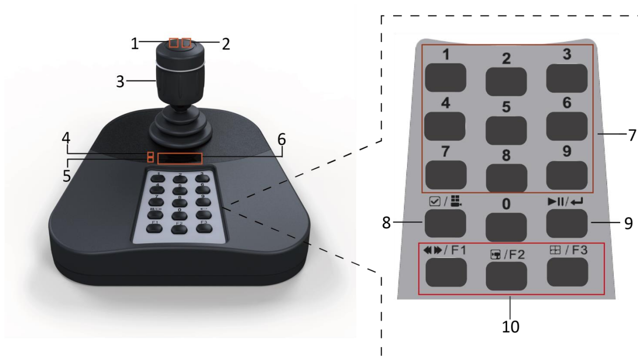
Рис. 1.2. Джойстик, функциональные кнопки и индикаторы
