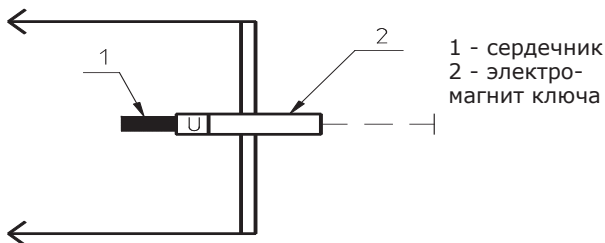
Рисунок Б.4 Принципиальная электрическая схема ключа
