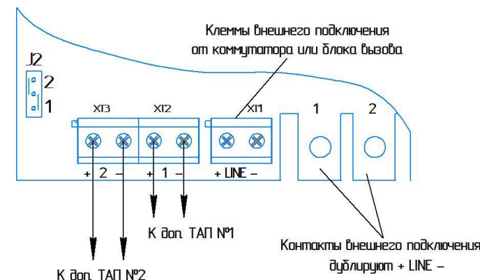
Рис. 2 Подключение ТАП КЛМ-2
