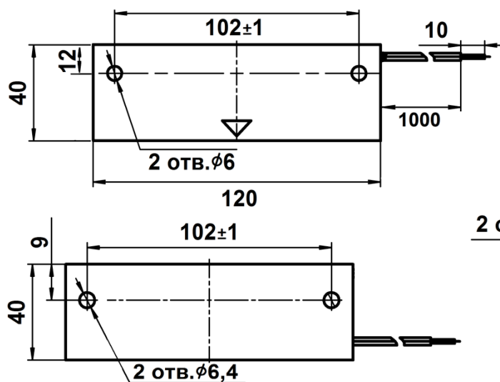
Блок датчика
