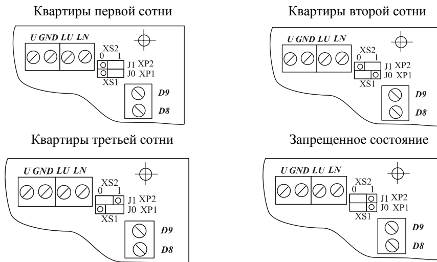
Рис.3 Положение джамперов XP1, XP2 и XP3 для различного диапазона квартир
