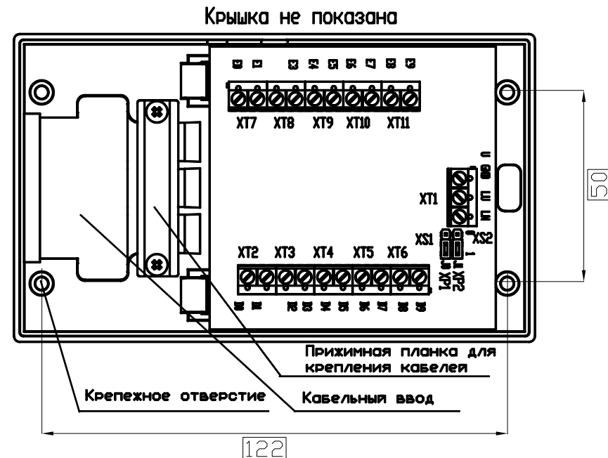
Рис. 2. Внешний вид KM100-7.3
