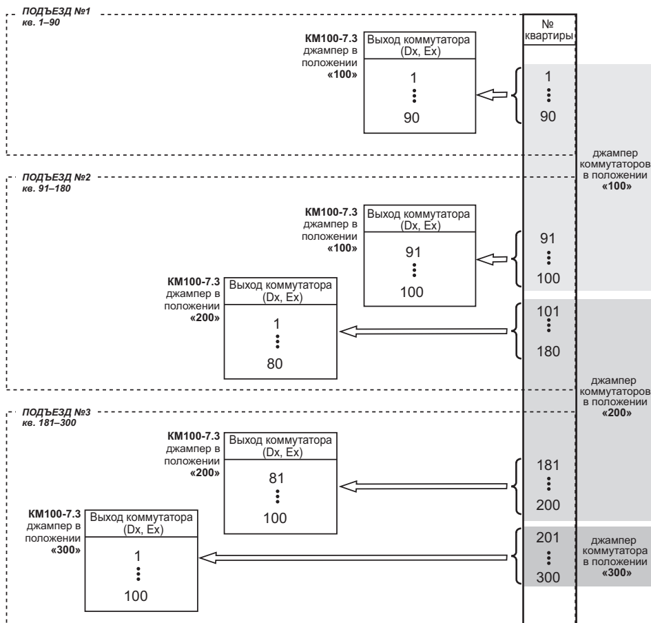
Рис.4 Пример схемы подключения подъездных коммутаторов КМ100-7.3
