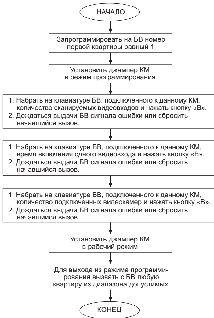
Рис.5 Алгоритм программирования управления видеокоммутацией
