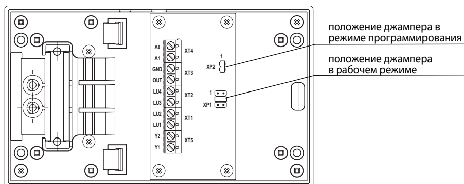
Рис.2 Вид КМ300-4.2 со снятой крышкой
