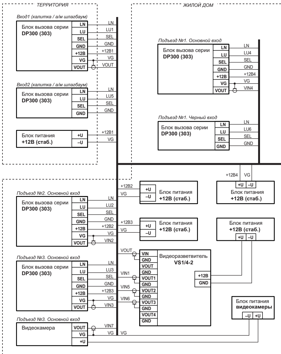
Рис.3 Схема подключения КМ300-4.2 к домофонному комплексу
