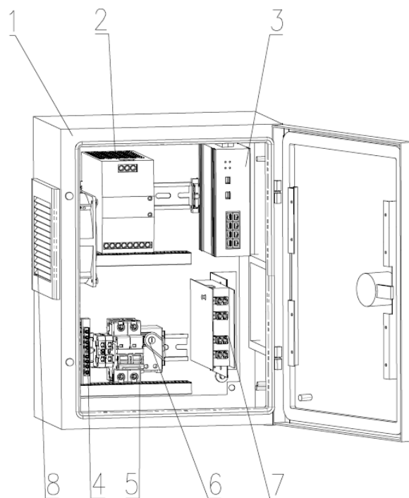
Рисунок 1 – Устройство изделия
