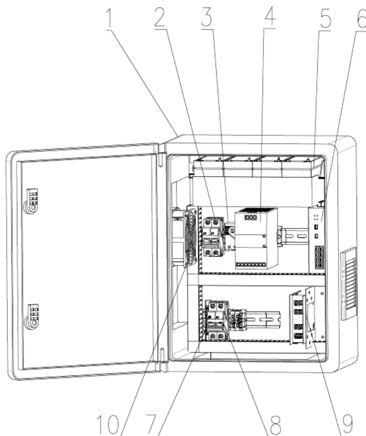
Рисунок 1 – Устройство изделия
