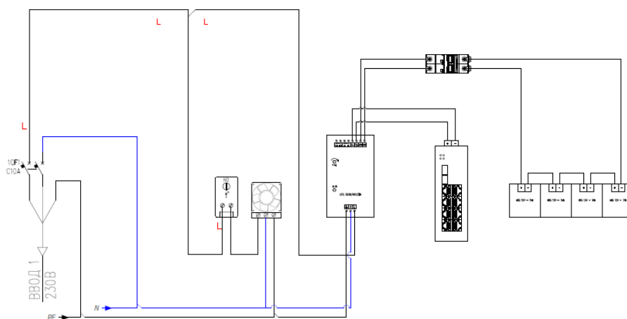
Рисунок 2 – Схема электрическая принципиальная
