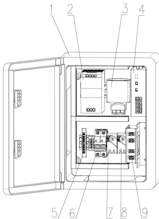
Рисунок 1 – Устройство изделия
