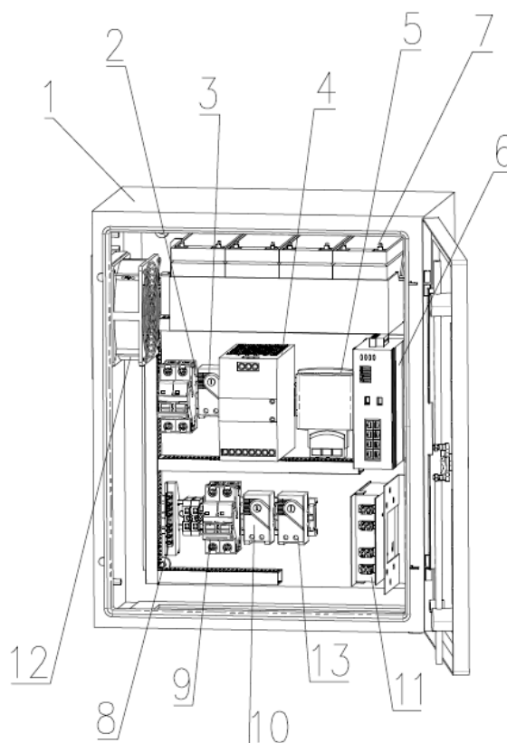
Рисунок 1 – Устройство изделия
