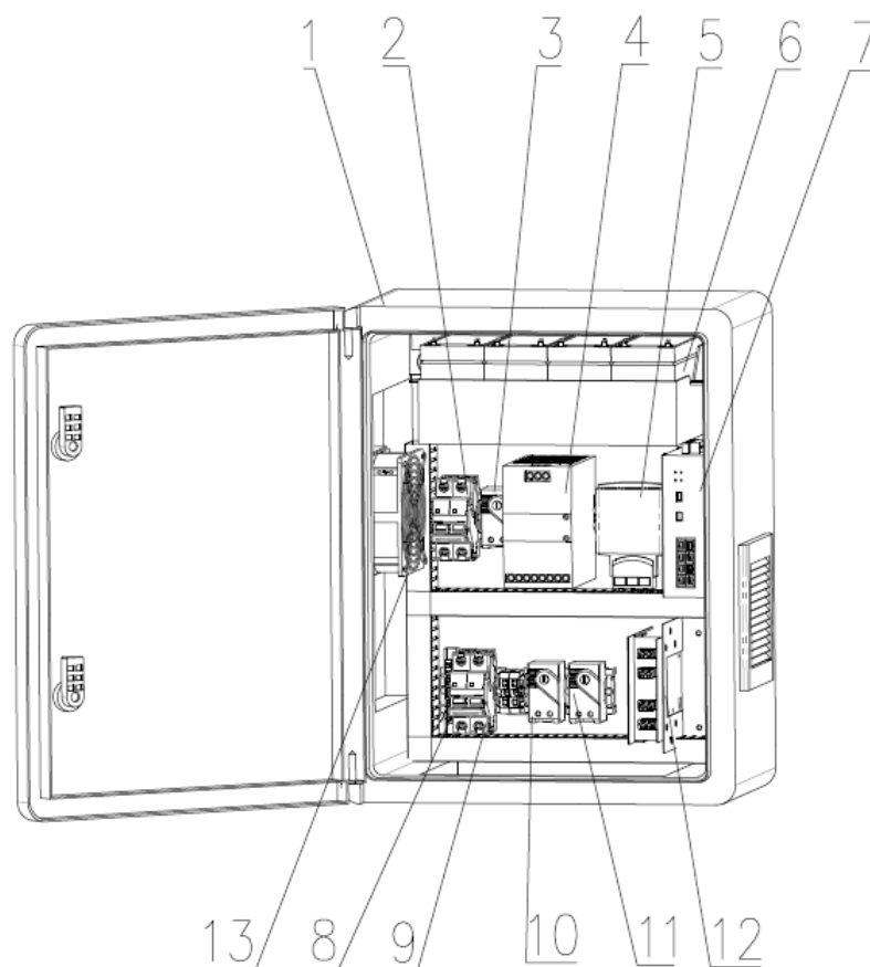
Рисунок 1 – Устройство изделия
