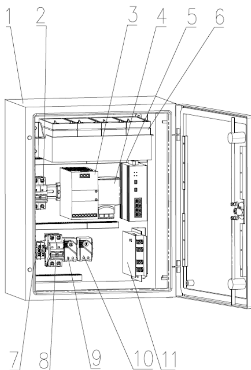
Рисунок 1 – Устройство изделия
