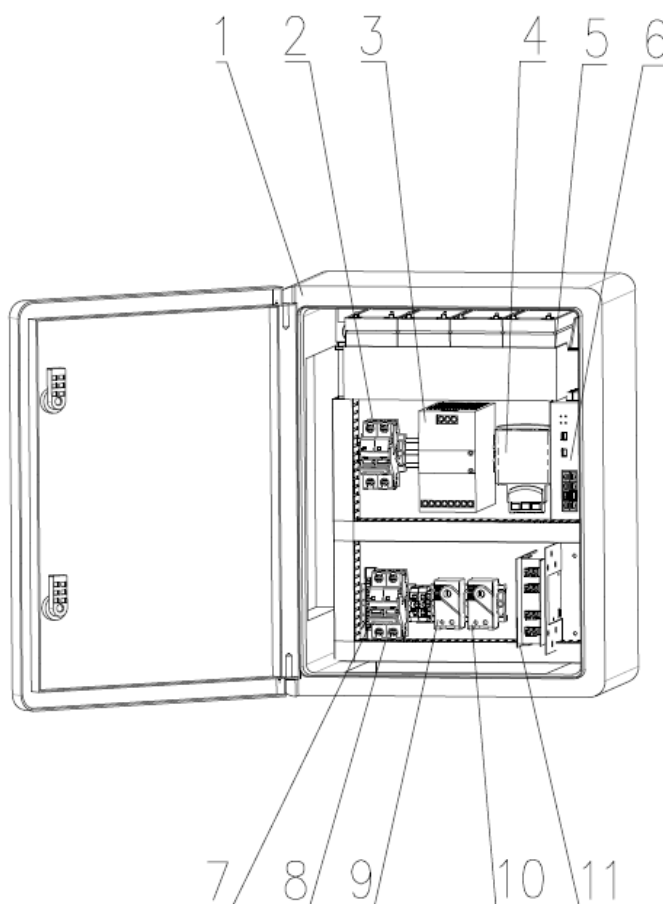
Рисунок 1 – Устройство изделия
