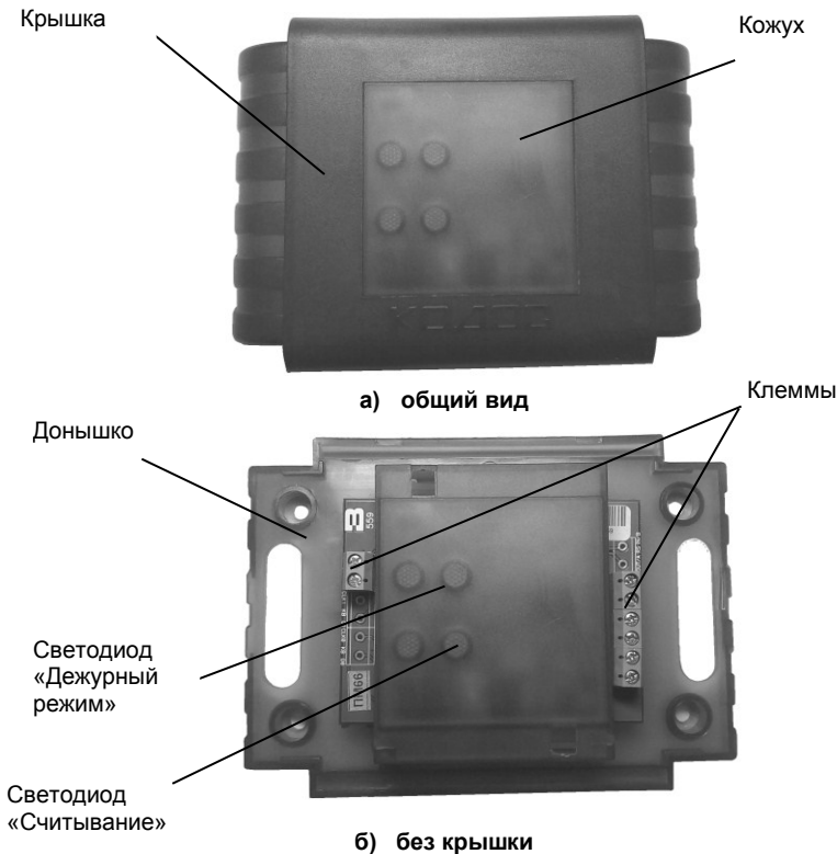
Рисунок 1 – Внешний вид адаптера
