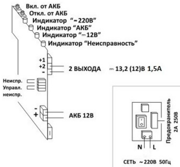
Рисунок 2 – Подключение контроллера
