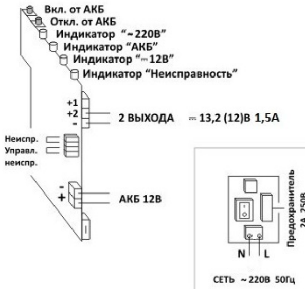
Рисунок 2 – Подключение контроллера
