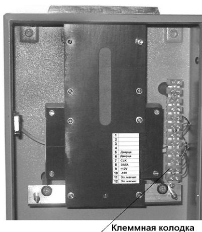
Рисунок 3 – Вид корпуса со снятой декоративной панелью
