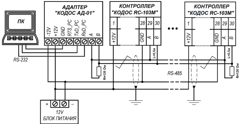
Рисунок 4а – Схема подключения контроллера к ПК с помощью адаптера «КОДОС АД-01»
