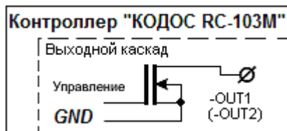
Рисунок 7 – Выходные каскады «-OUT1» и «-OUT2»
