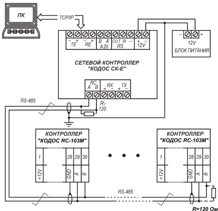
Рисунок 46 – Схема подключения контроллера к ПК с помощью сетевого контроллера «КОДОС СК-Е»
