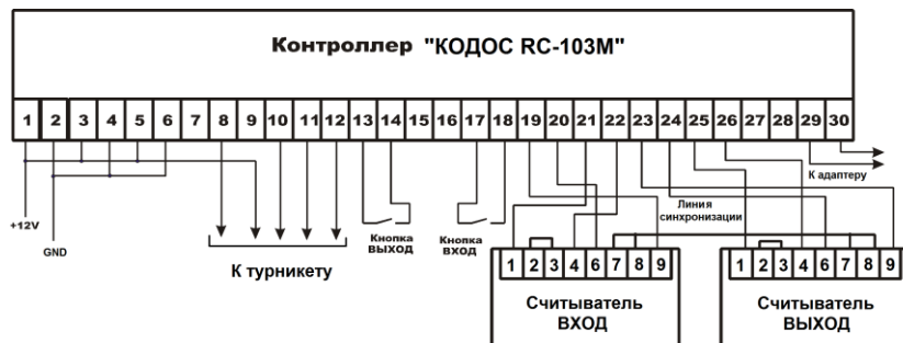
Рисунок 11 – Схема подключения (вариант 2)
