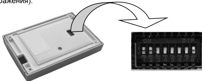
Рисунок 22 – DIP-переключатели контроллера
