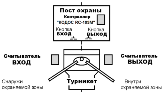
Рисунок 10 – Два внешних считывателя, контроллер в режиме работы с внешними считывателями серии «КОДОС RD»
