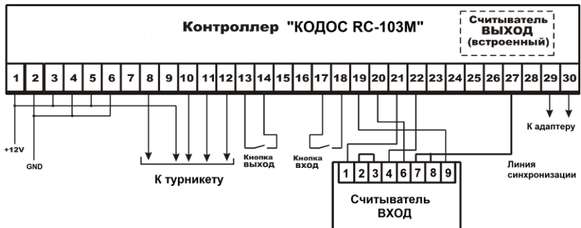
Рисунок 9 – Схема подключения (вариант 1)
