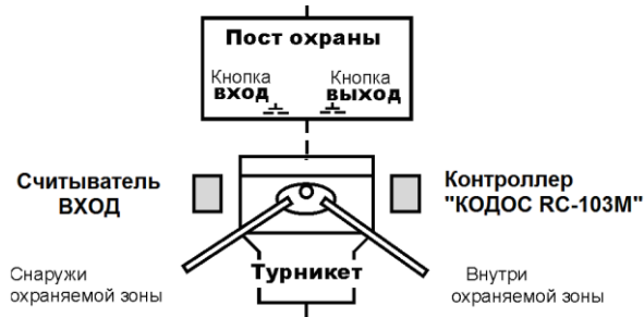
Рисунок 8 – Один внешний считыватель серии «КОДОС RD», контроллер в режиме работы со встроенным считывателем
