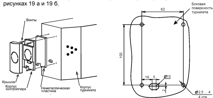
Рисунок 19 – Монтаж контроллера на боковой стороне турникетов «РостЕвроСтрой» серии Тх (за исключением Т83, Т283)
