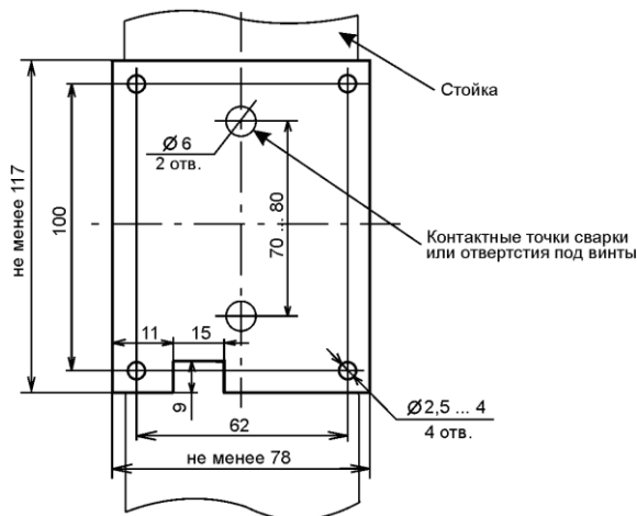
Рисунок 21 – Крепление контроллера
