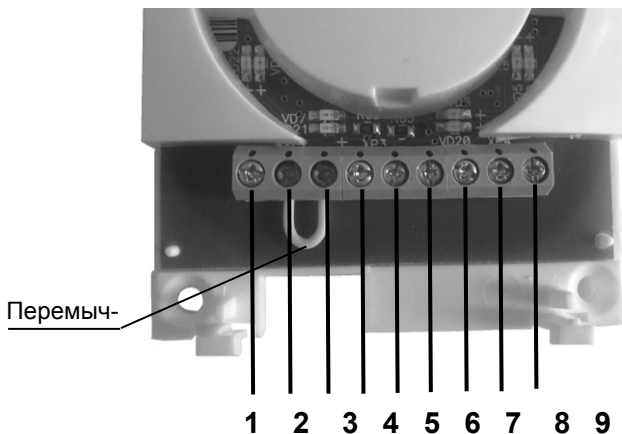
Рисунок 3 – Клеммы считывателя
