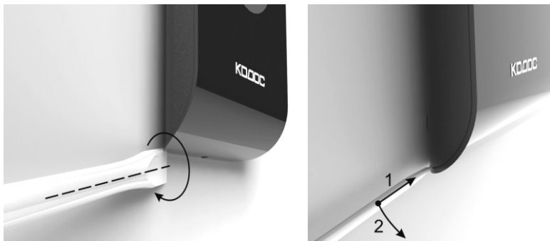
Рисунок 2.3 – Демонтаж крышки считывателя
