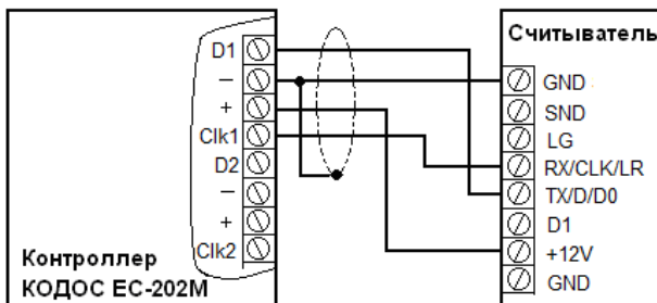
Рисунок 2.5 – Пример схемы экранирования
