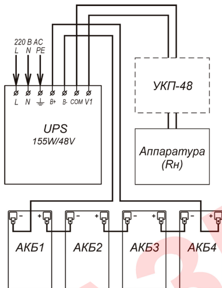
Рисунок 2 – Схема электрическая принципиальная
