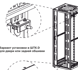
Вариант установки в ШТК-Э для боковой обшивки
