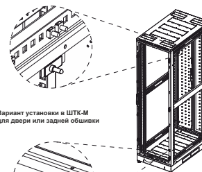
Вариант установки в ШТК-М для боковой обшивки
