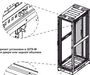
Вариант установки в ШТК-М для боковой обшивки
