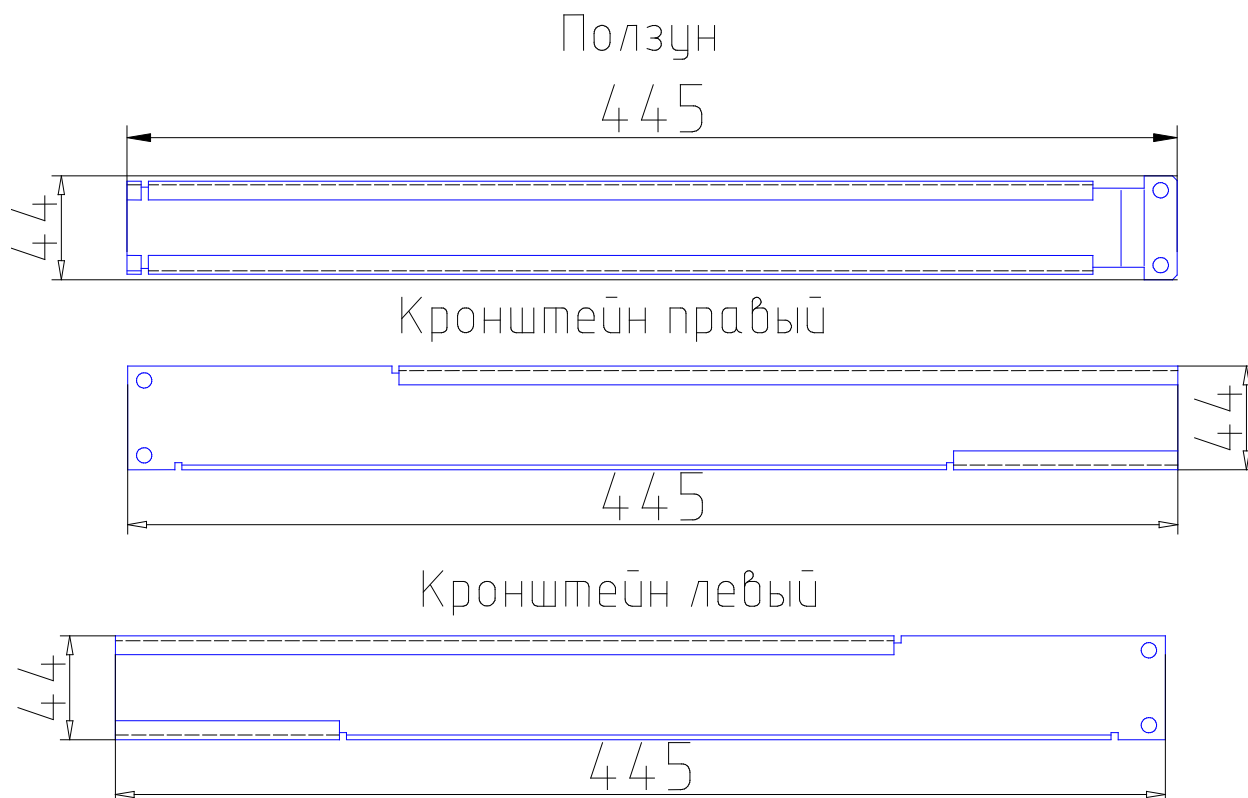
Рисунок 1 – Состав изделия и его габаритные размеры Комплектность изделия приведена в таблице 1.
