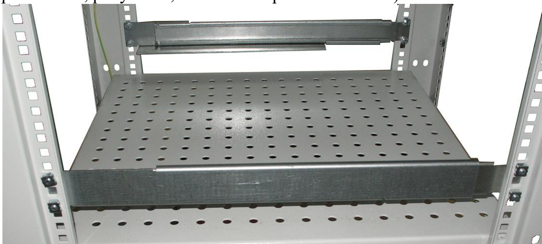
Рисунок 2 – Вид на крепление кронштейнов в стойке сбоку
