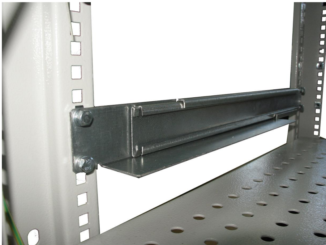
Рисунок 4 – Вид на кронштейн и поддерживающий уголок
