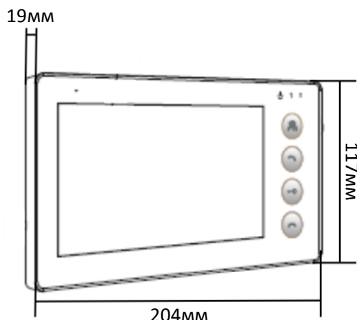
Видеодомофон
