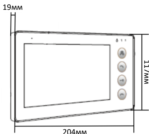
Видеодомофон
