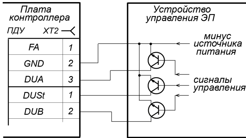
Рисунок 9. Управление ЭП схемой с открытым коллекторным выходом
