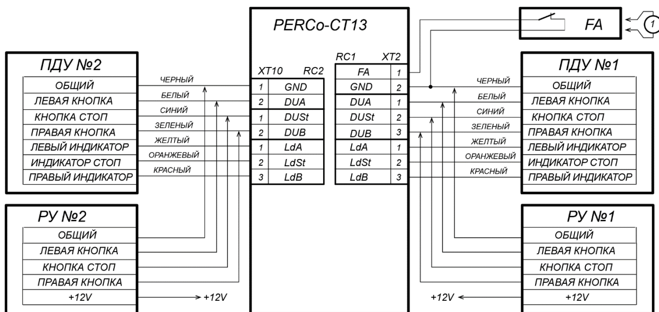
ПДУ (РУ) №1 - для управления ЭП PERCo-KT02.9B, ПДУ (РУ) №2 - для управления ИУ №2 (дополнительным турникетом, калиткой, шлагбаумом) ① – провод-перемычка, устанавливается при отсутствии устройства FA
