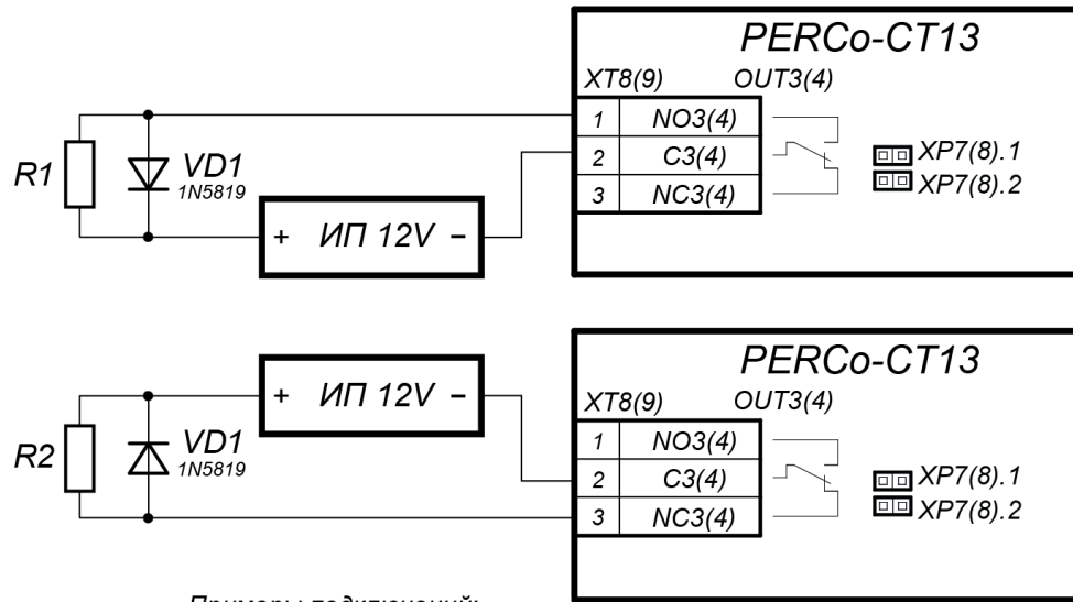
Рисунок 24. Схема подключений дополнительного оборудования к релейным выходам контроллера
