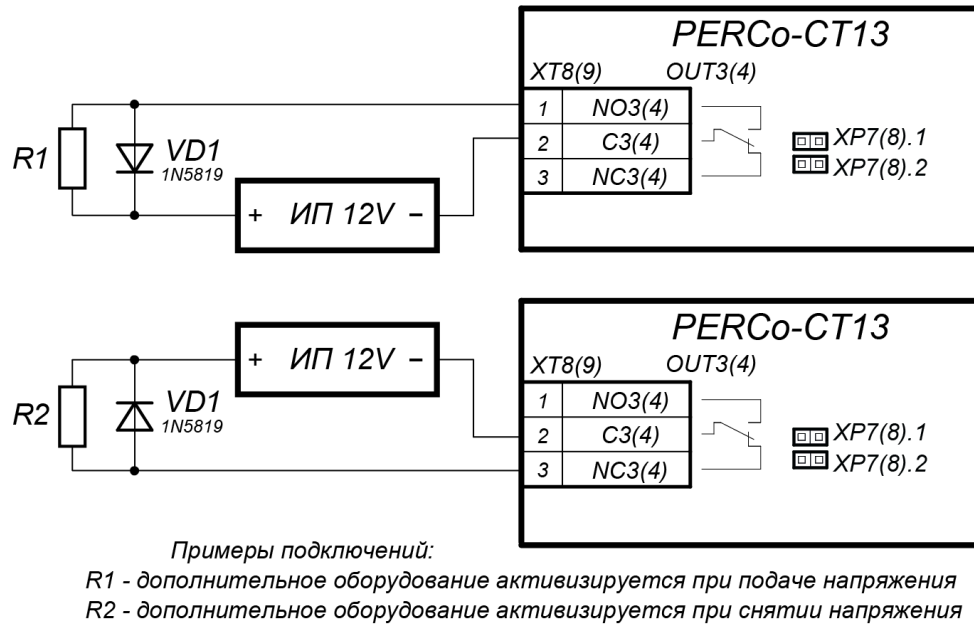
Рисунок 24. Схема подключений дополнительного оборудования к релейным выходам контроллера
