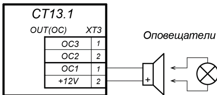
Рисунок 22. Схема подключений дополнительного оборудования к выходам контроллера типа «Открытый коллектор»
