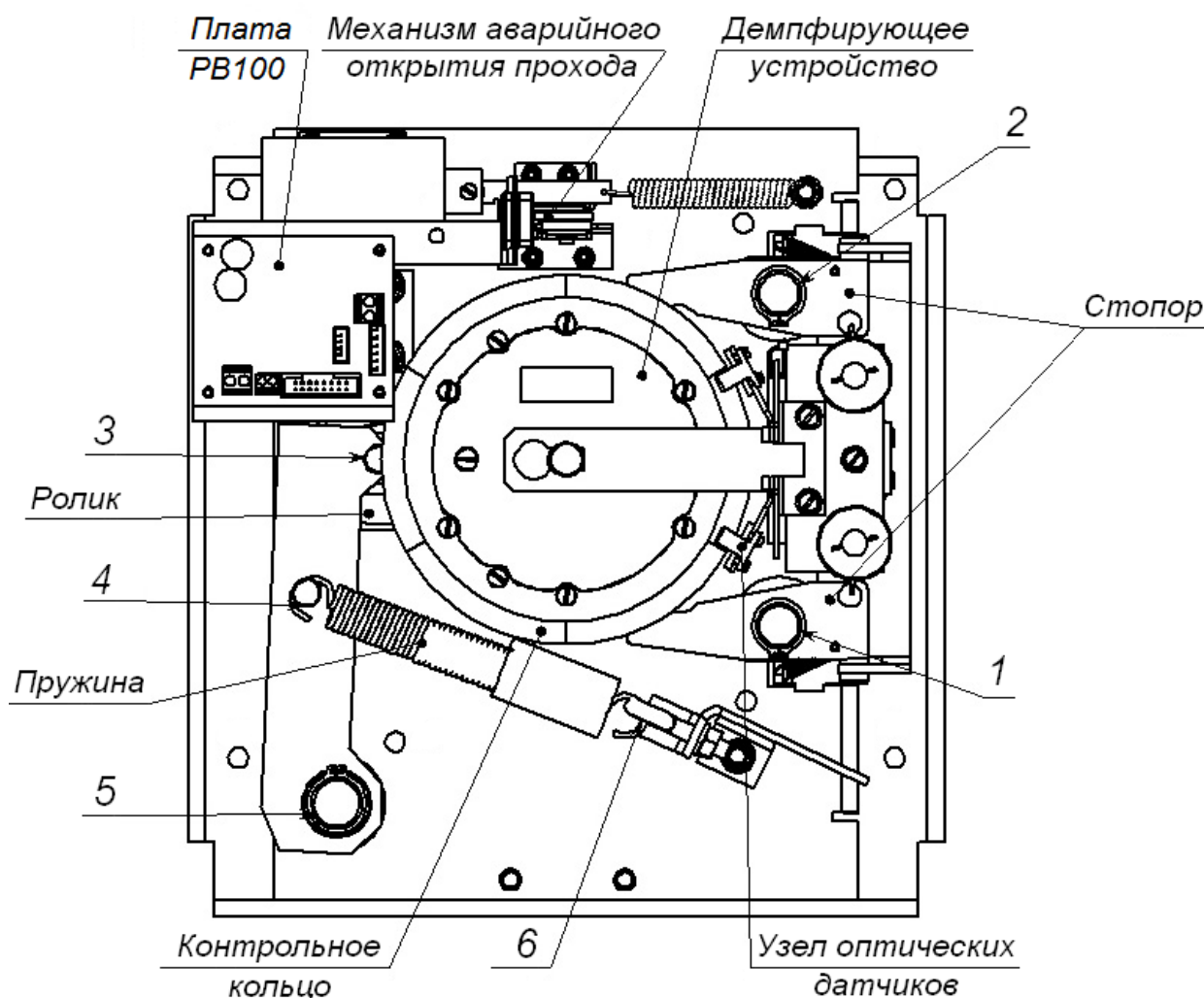
Рисунок 24. Расположение внутренних деталей и узлов стойки ЭП
