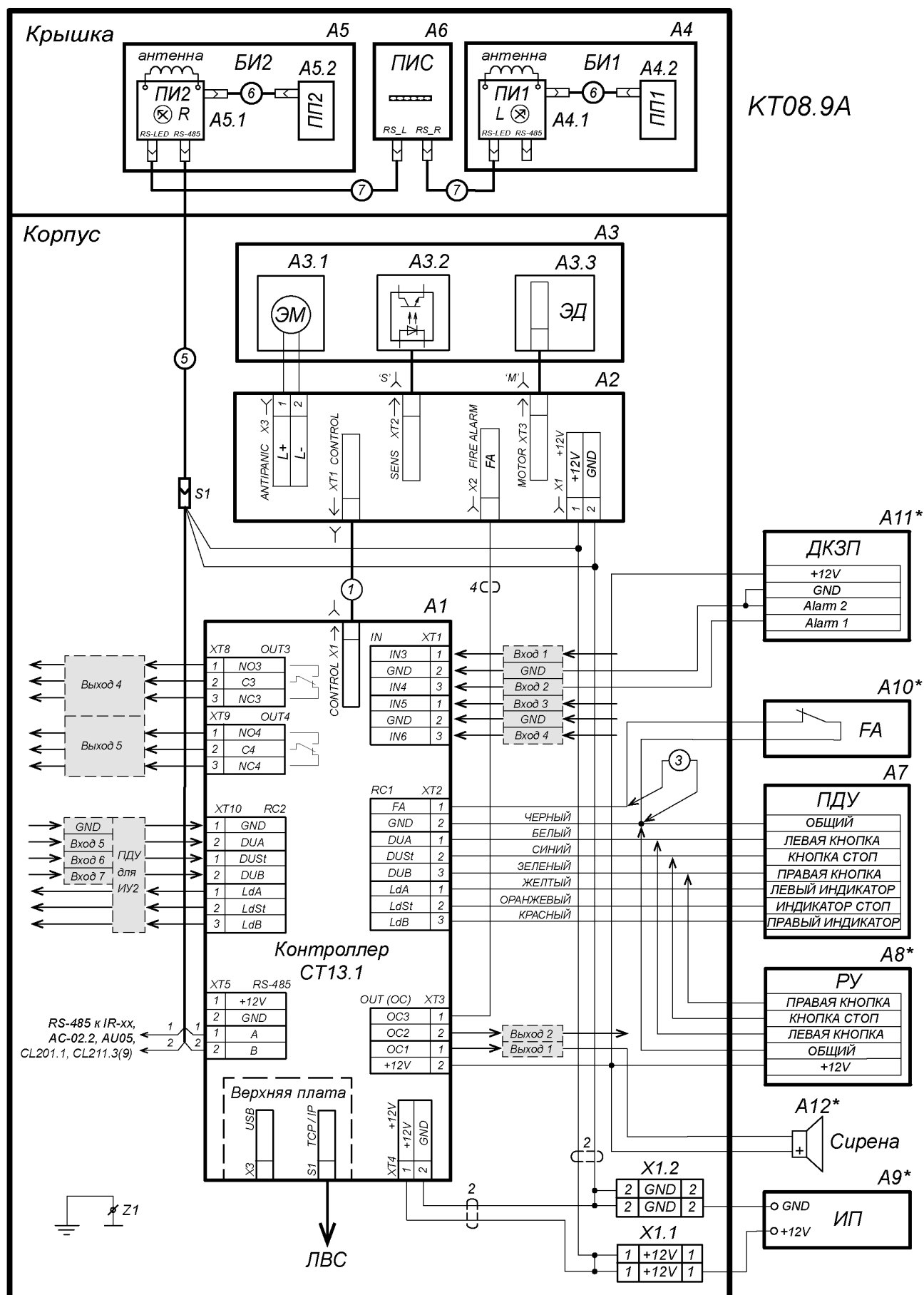
Рисунок 13. Схема подключения ЭП и дополнительного оборудования
