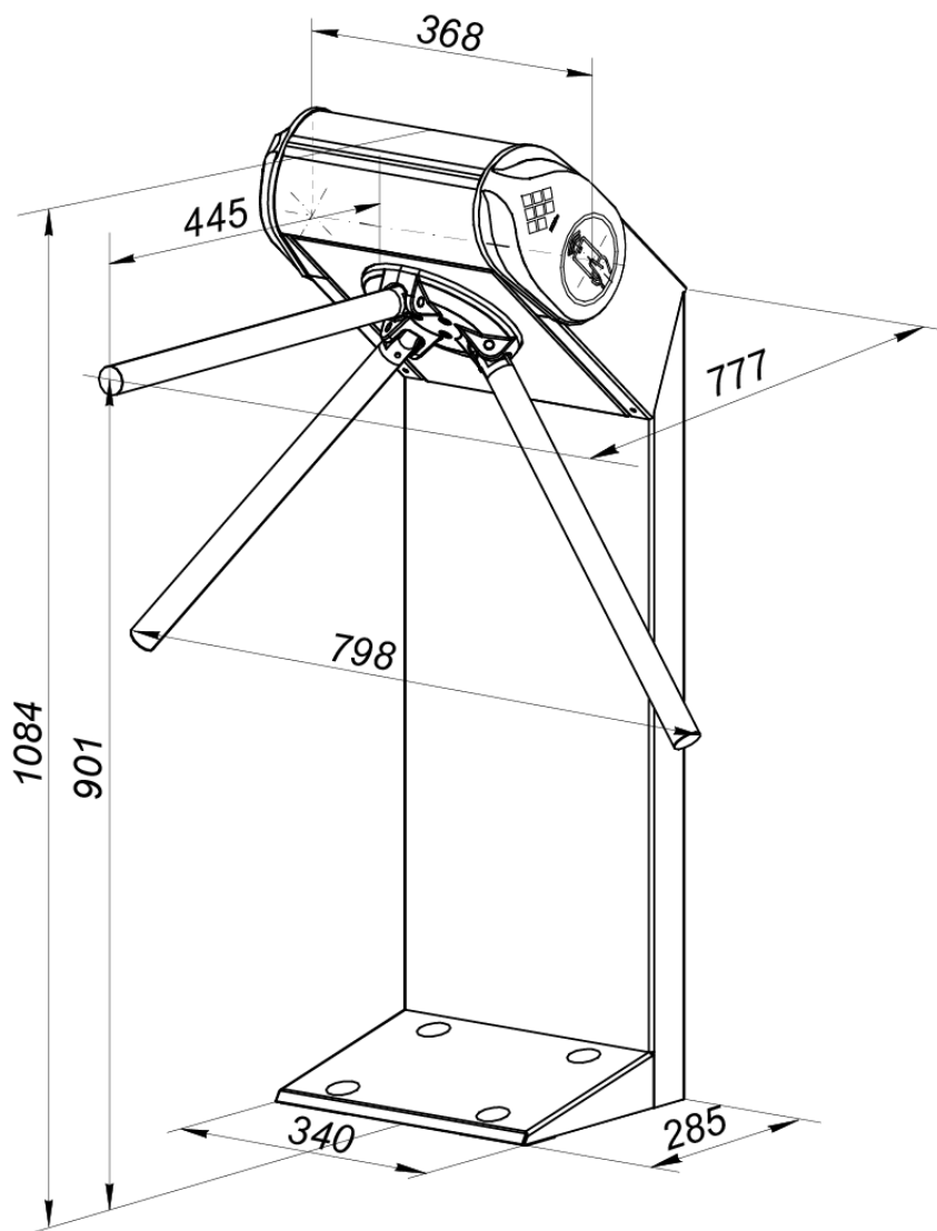
Рисунок 1. Габаритные размеры ЭП
