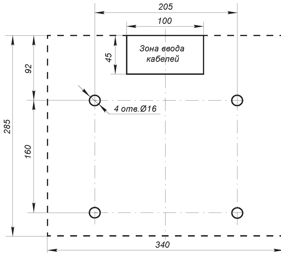
Рисунок 10. Разметка отверстий в полу под крепление стойки ЭП (пунктиром показаны габариты основания) 1
