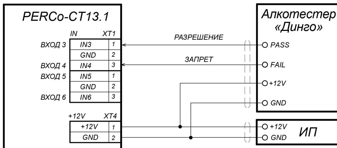
Рисунок 28. Схема подключения алкотестера «Динго В-02» (ООО СИМС-2)
