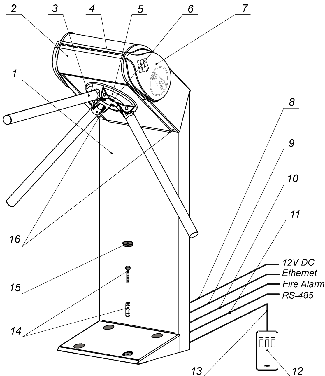
Рисунок 2. Устройство ЭП:
