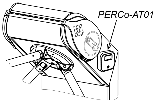
Рисунок 31. Вариант установки пирометра PERCo-AT01 на крышку ЭП
