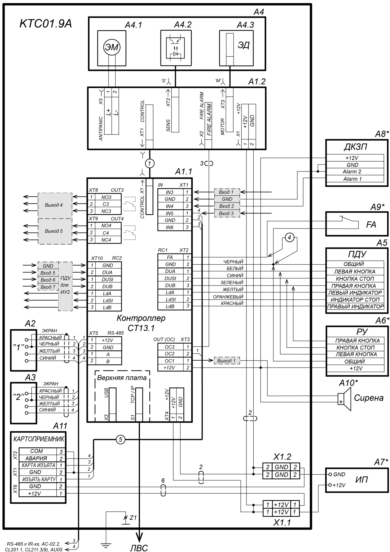
Рисунок 14. Схема подключения ЭП и дополнительного оборудования
