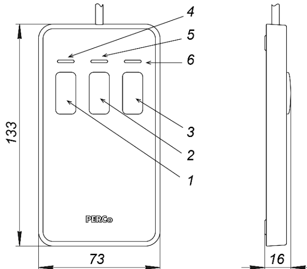
Рисунок 5. Общий вид и габаритные размеры ПДУ
