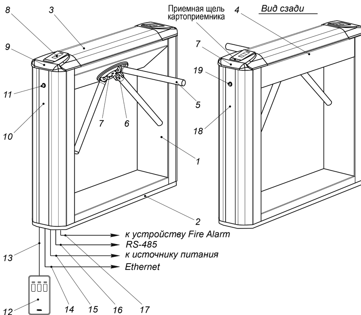
Рисунок 2. Устройство ЭП
