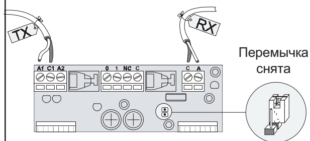
ПОДКЛЮЧЕНИЕ 1 ПАРЫ ФОТОЭЛЕМЕНТОВ
