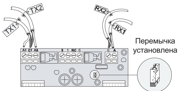
ПОДКЛЮЧЕНИЕ 2 ПАР ФОТОЭЛЕМЕНТОВ
