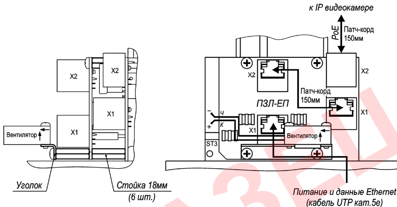
Рис.2 Установка платы ПЗЛ-ЕП в гермобоксы ТГБ-4Г Ex PoE+, ТГБ-8Г Ex PoE+, ТГБ-9 PoE+
