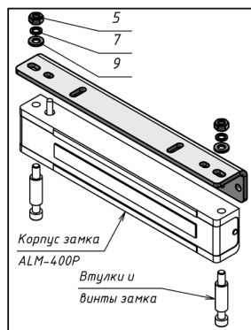
Рисунок 1 – Установка корпуса и якоря замка с комплектом МК 300-400-IN
