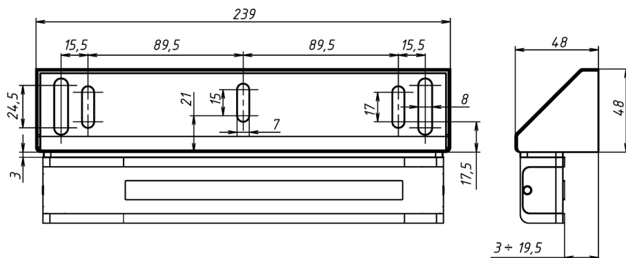
Рисунок 2 – Габаритный чертеж
