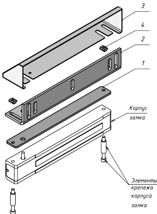
Рисунок 1 – Комплект поставки
