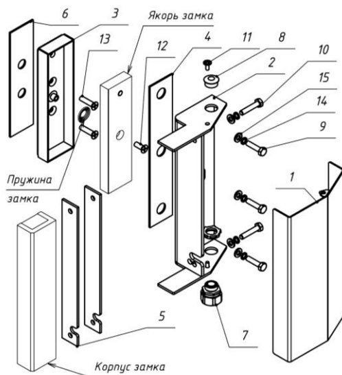
Рисунок 1 – Комплект МК 350FB-GP.
