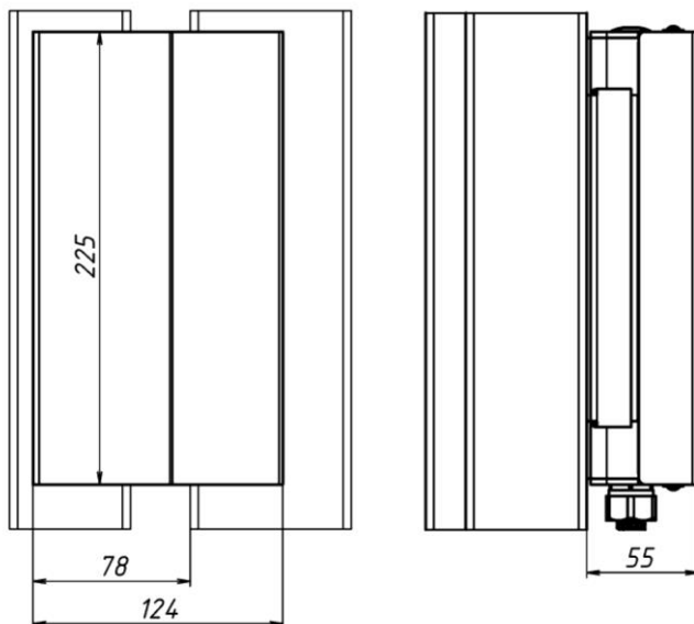
Рисунок 5 – Габариты комплекта в проеме двери
