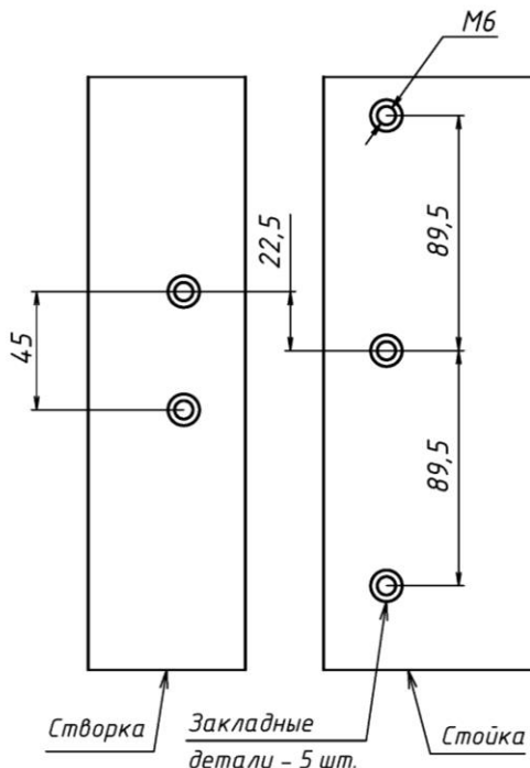
Рисунок 2 – Установка закладных деталей
