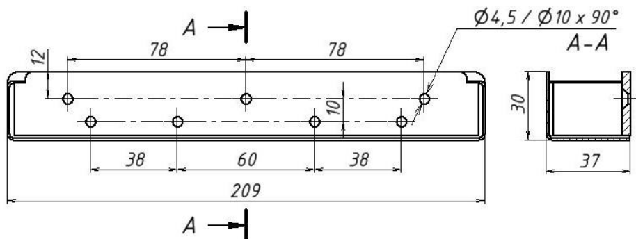
Рисунок 2 – Габаритно-установочные размеры комплекта МК 700S
