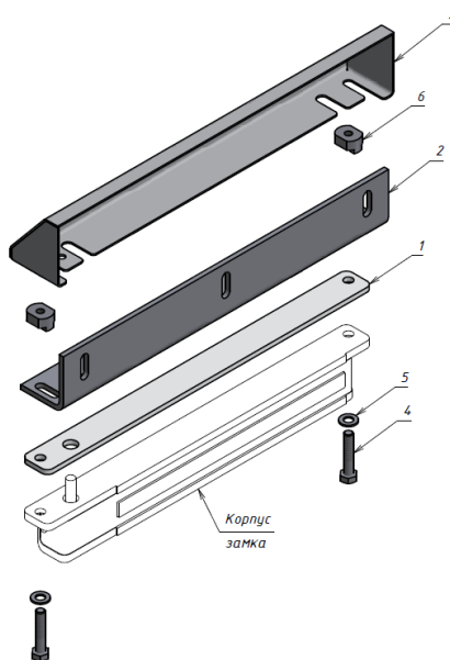
Рисунок 1 – Комплект поставки
