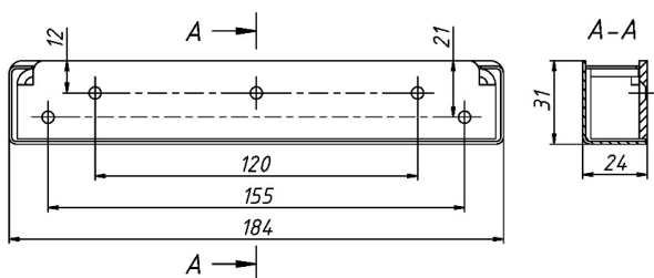
Рисунок 2 – Габаритно-установочные размеры комплекта МК AL-250S
