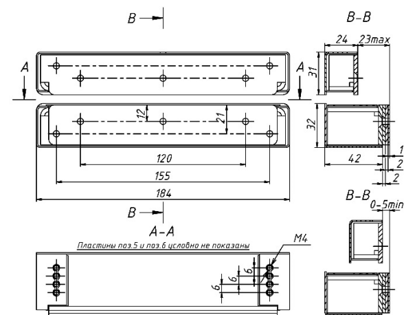
Рисунок 2 – Габаритно-установочные размеры комплекта МК AL-250SM-Shift
