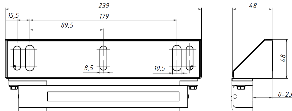
Рисунок 2 – Габаритный чертеж
