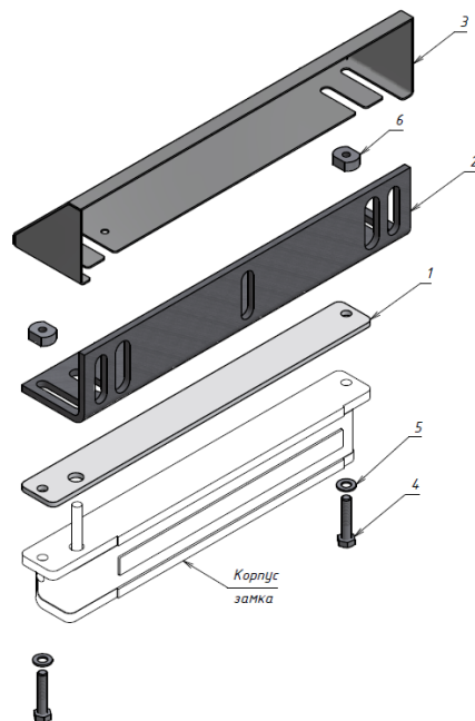
Рисунок 1 – Комплект поставки
