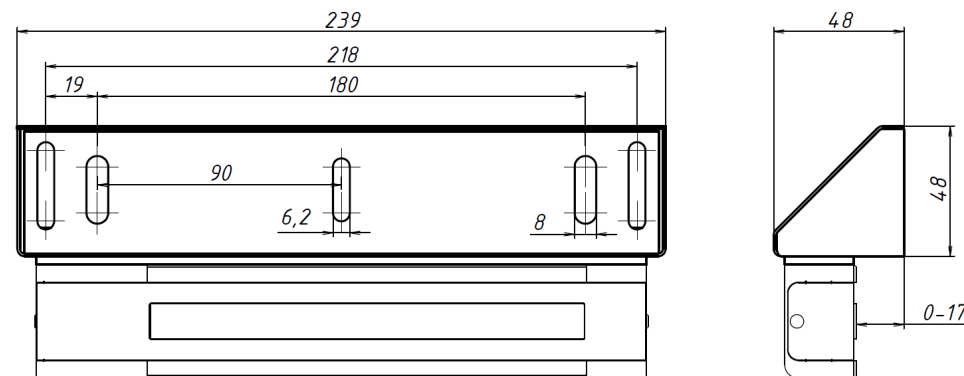
Рисунок 2 – Габаритный чертеж
